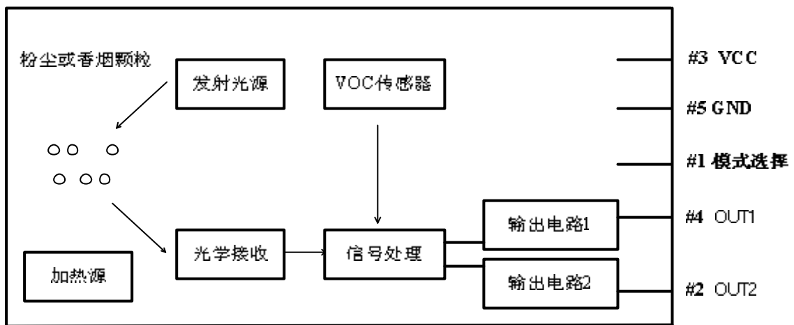
图2：原理示意1
