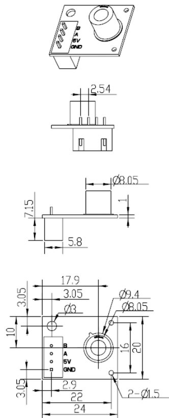
图 1：模组结构图
