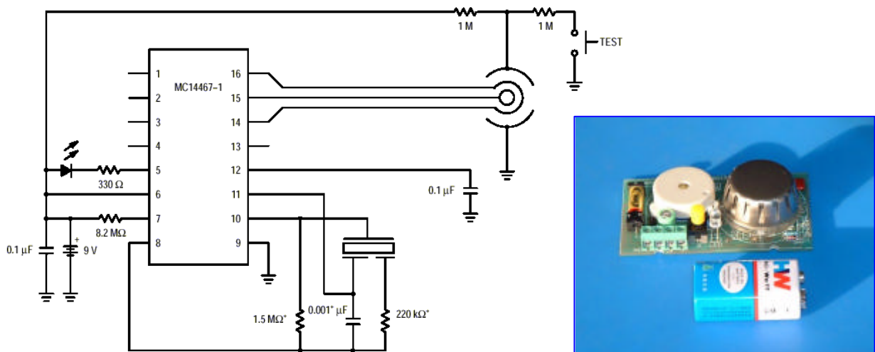
采用 MC14468 的烟雾探测器电原理图
