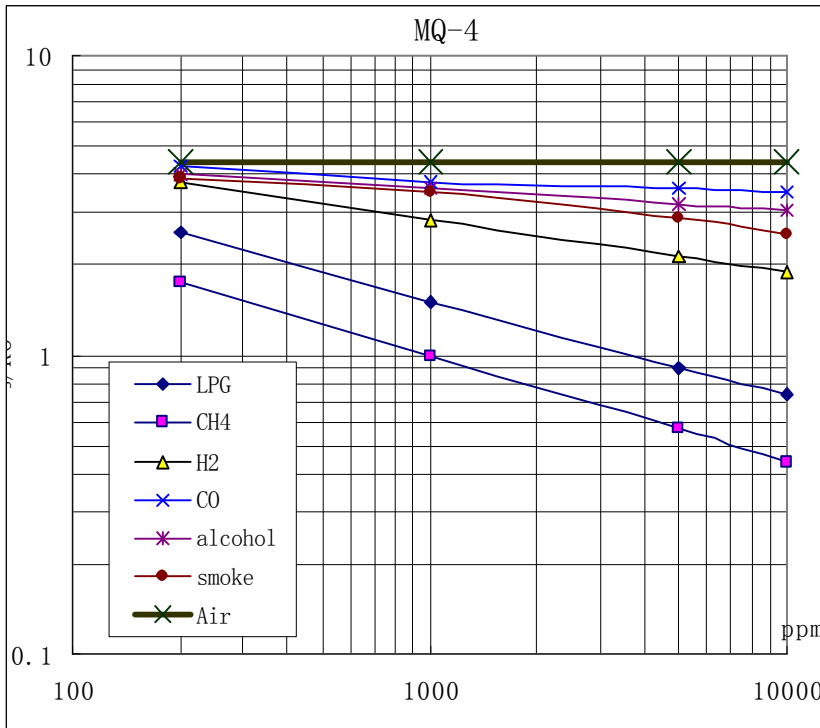
图 3 MQ-4型气敏元件的灵敏度特性
