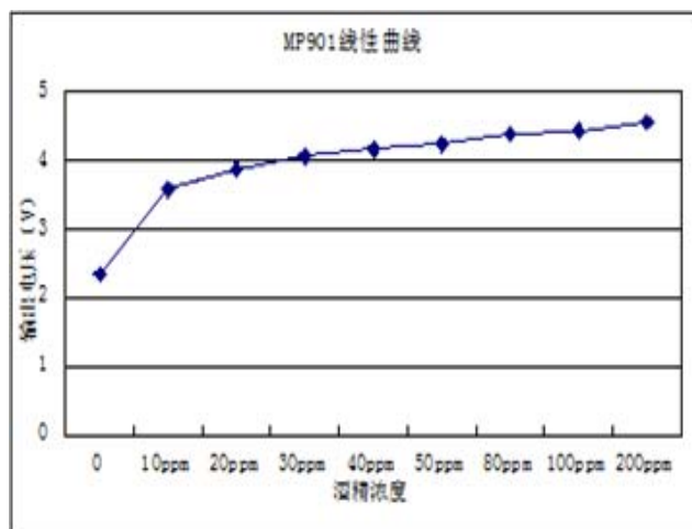
图6：传感器线性曲线
