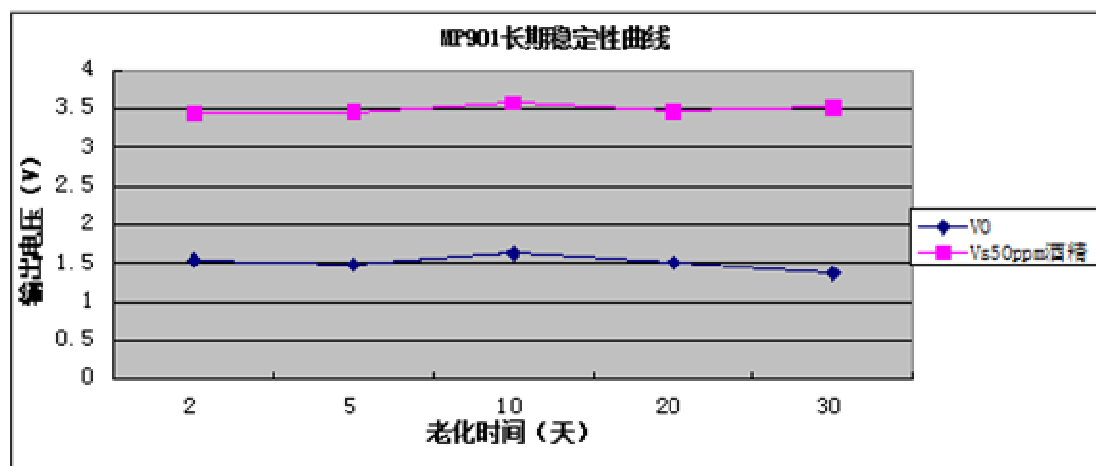
图 7: 长期稳定性曲线
