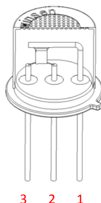
图 8： 管脚示意图
