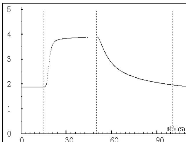
图5：响应恢复曲线
