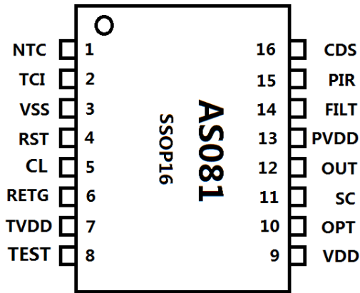
AS081 SSOP16
